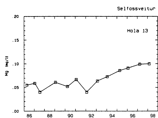
Mynd 34. Styrkur magnesíums í vatni úr holu 13
