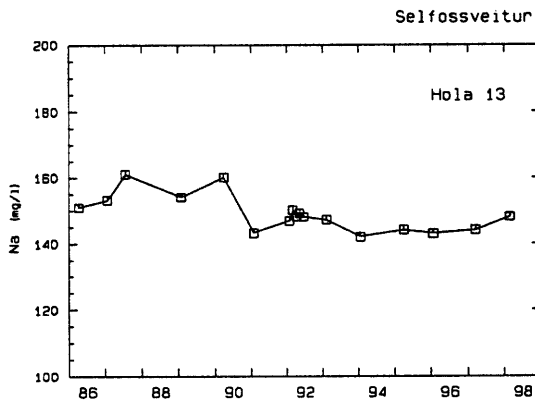
Mynd 31. Styrkur natríums í vatni úr holu 13
