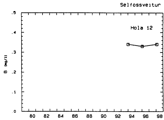
Mynd 26. Styrkur bórs í vatni úr holu 12
