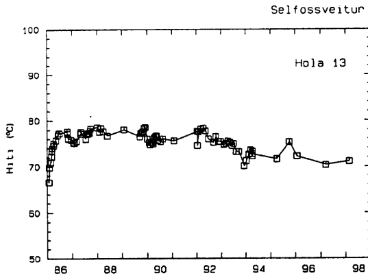
Mynd 29. Hiti vatns úr holu 13
