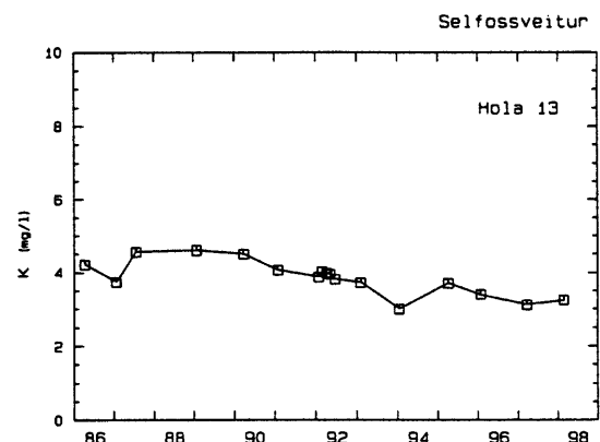
Mynd 32. Styrkur kalíums í vatni úr holu 13
