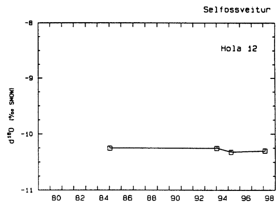
Mynd 28. Súrefnissamsætur í vatni úr holu 12
