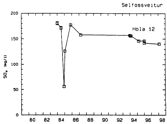
Mynd 24. Styrkur súlfats í vatni úr holu 12
