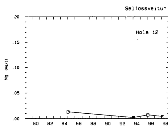
Mynd 22. Styrkur magnesíums í vatni úr hólú 12
