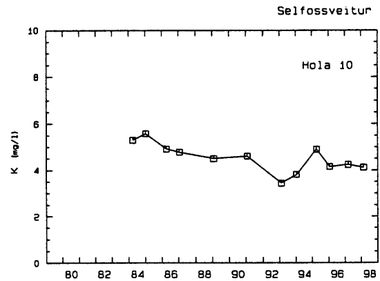
Mynd 8. Styrkur kalíúms í vatni úr hól 10
