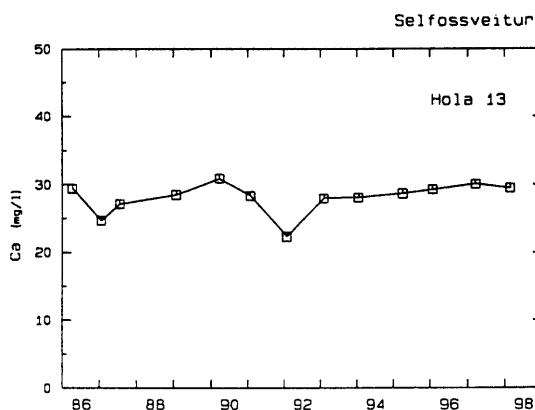
Mynd 33. Styrkur kalsíums í vatni úr holu 13
