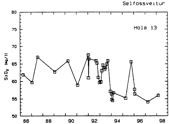
Mynd 30. Styrkur kísils í vatni úr holu 13
