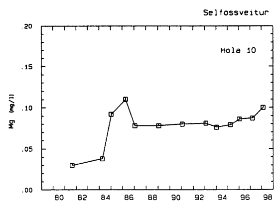
Mynd 10. Styrkur magnesíúms í vatni úr hól 10
