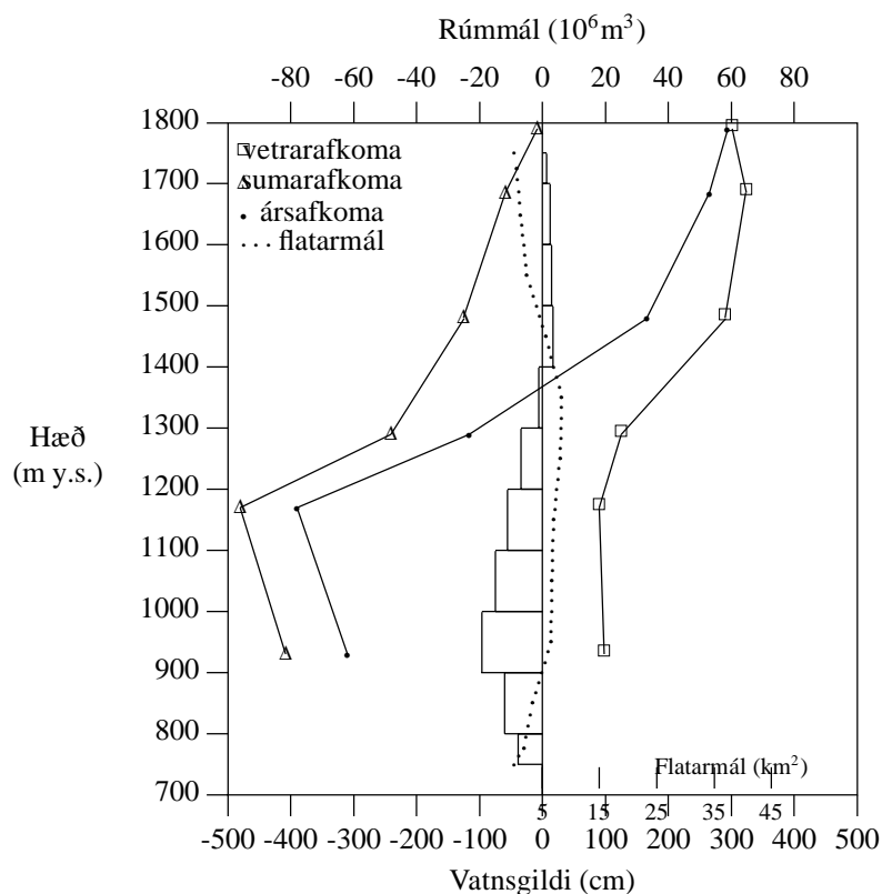
Mynd V-12. Línurit yfir afkomu Blágnjúpjökuls í Hofsjökli 1995-1996.
