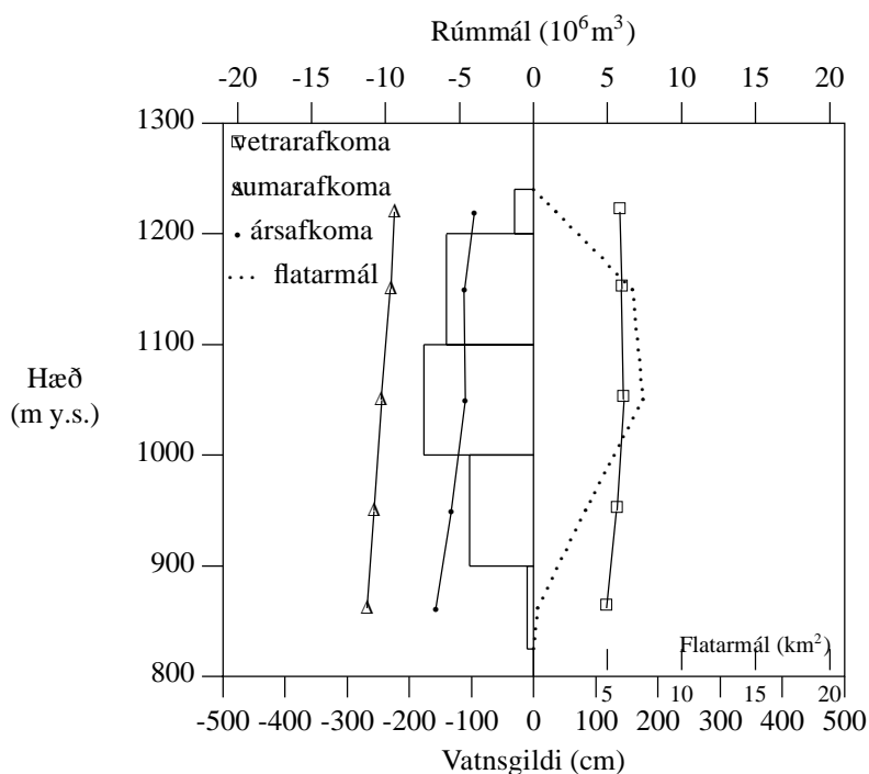
Mynd V-21. Línurit yfir afkomu Þrándarjökuls 1994-1995.
