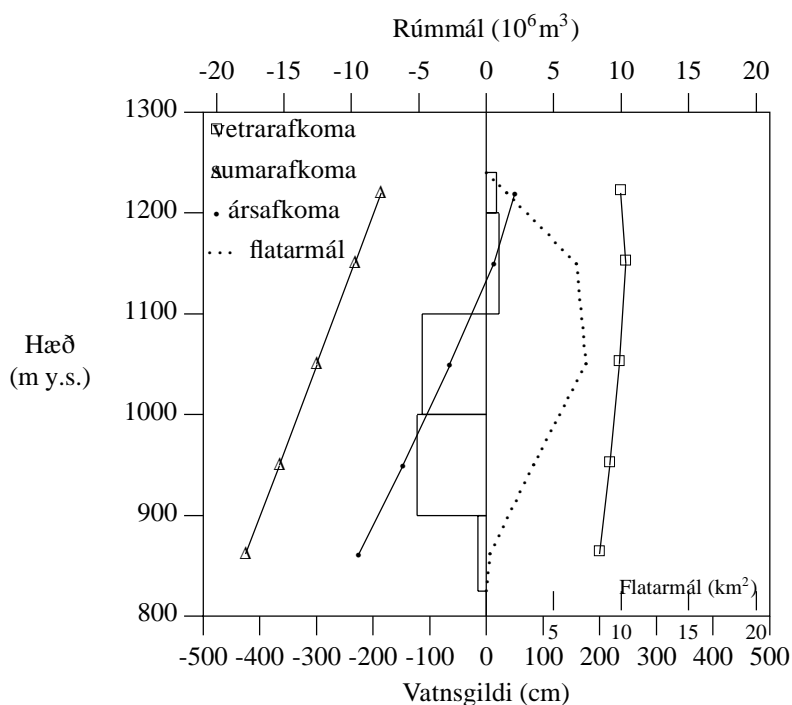
Mynd V-22. Línurit yfir afkomu Þrándarjökuls 1995-1996.
