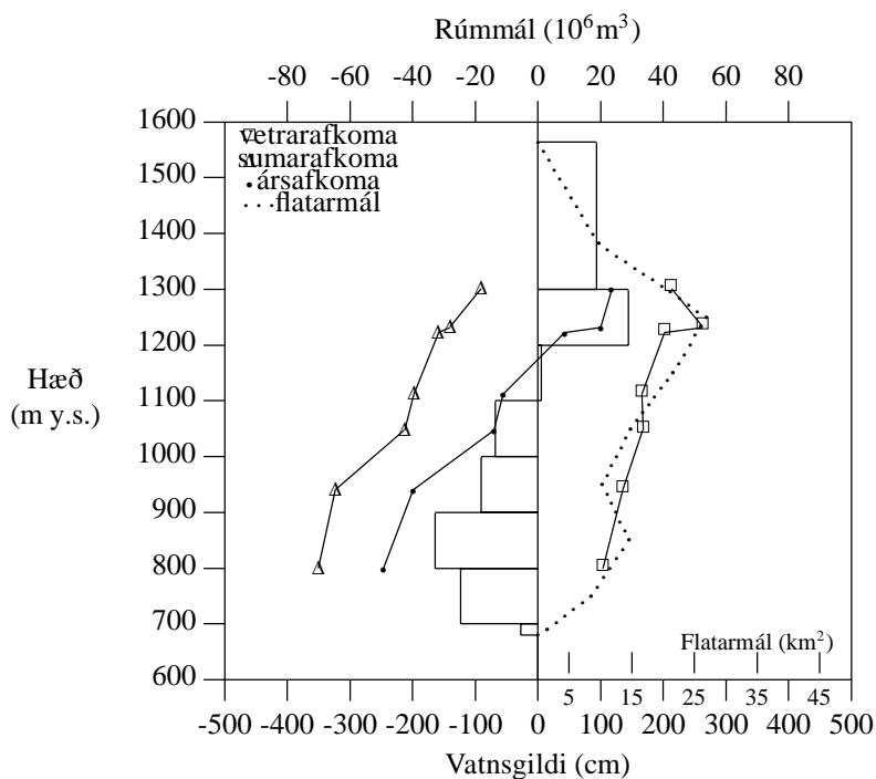
Mynd V-18. Línurit yfir afkomu Eyjabakkajökuls í Vatnajökli 1994-1995.
