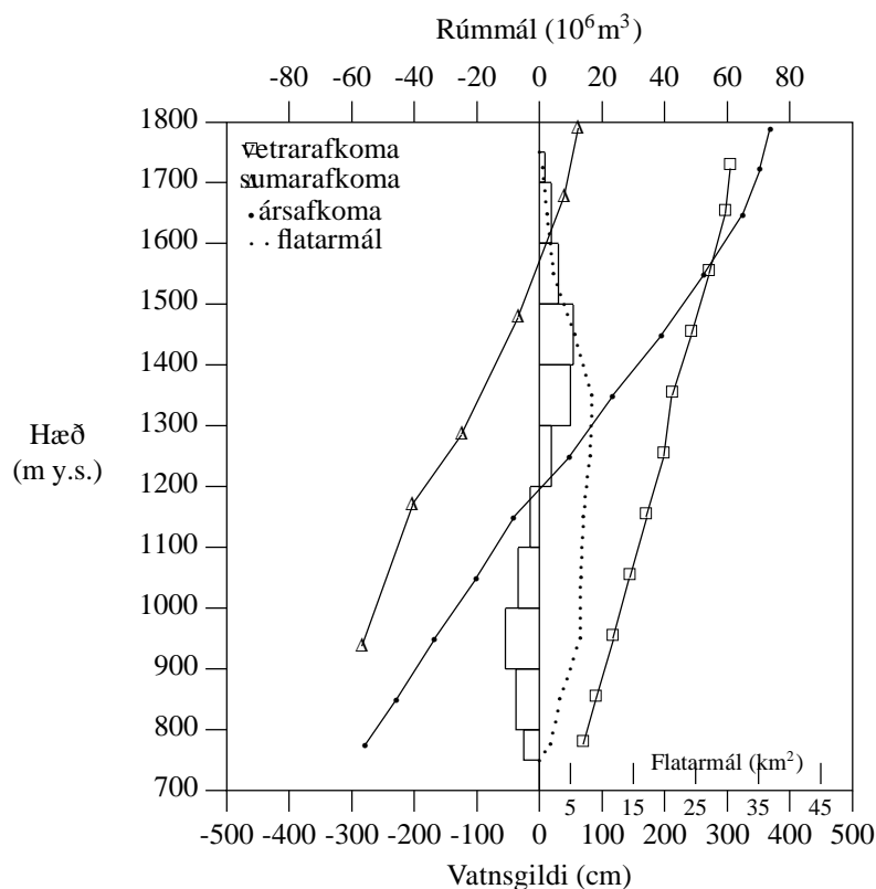
Mynd V-3. Línurit yfir afkomu Blágnípujökuls í Hofsjökli 1992-1993.
