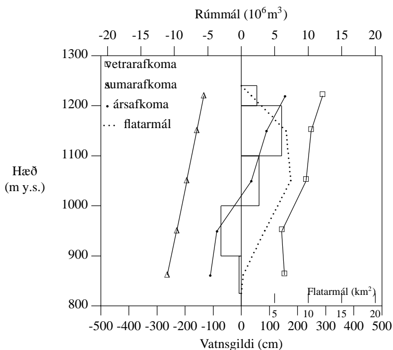
Mynd V-20. Línurit yfir afkomu Þrándarjökuls 1993-1994.
