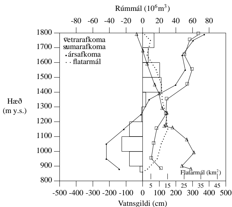
Mynd V-4. Línurit yfir afkomu Sátujökuls í Hofsjökli 1993-1994.
