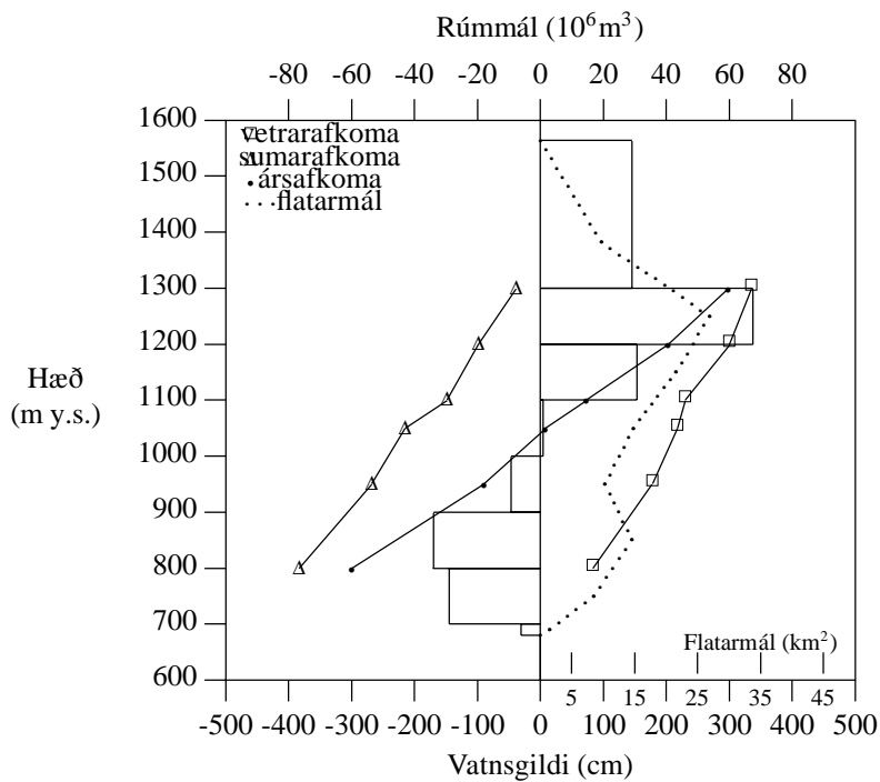
Mynd V-17. Línurit yfir afkomu Eyjabakkajökuls í Vatnajökli 1993-1994.
