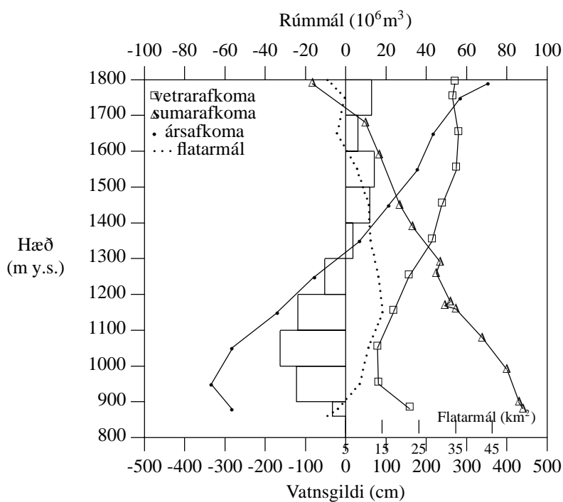
Mynd V-7. Línurit yfir afkomu Sátujökuls í Hofsjökli 1994-1995.
