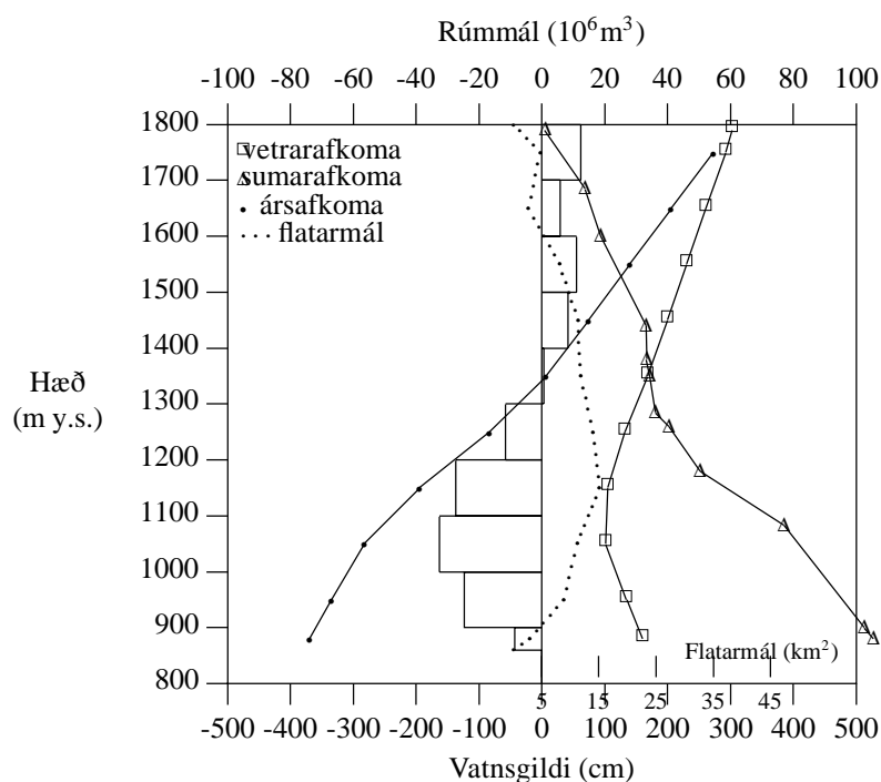
Mynd V-10. Línurit yfir afkomu Sátujökuls í Hofsjökli 1995-1996.
