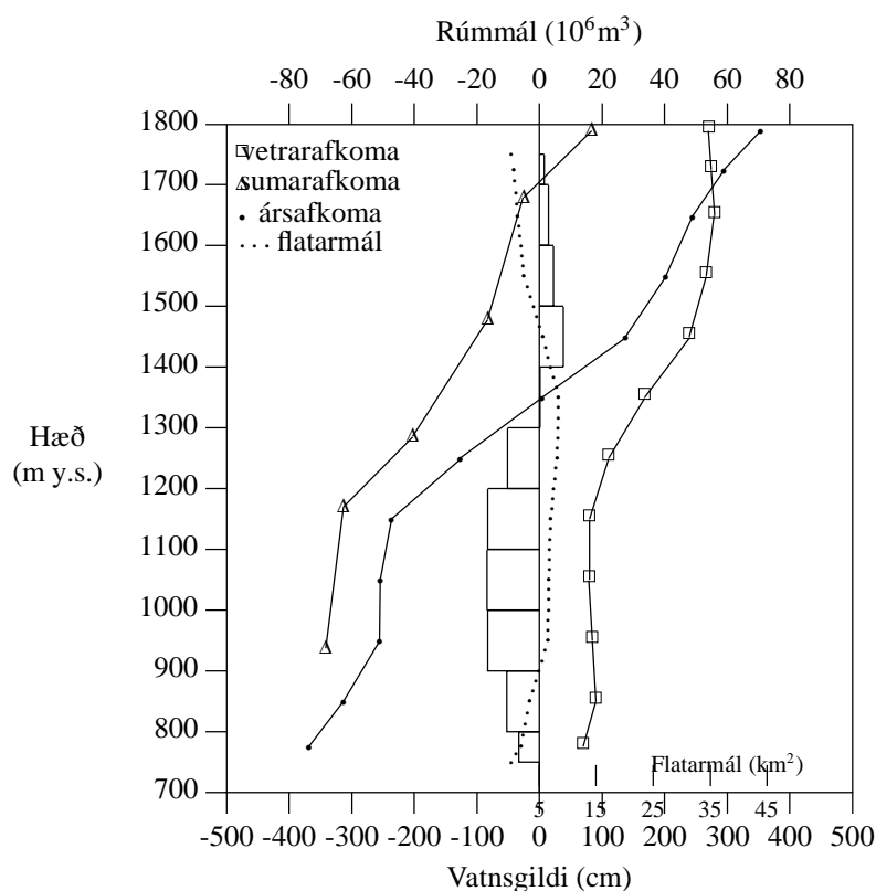
Mynd V-9. Línurit yfir afkomu Blágnípujökuls í Hofsjökli 1994-1995.
