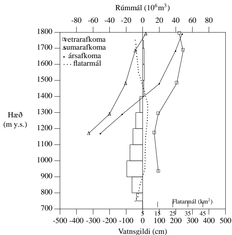
Mynd V-15. Línurit yfir afkomu Blágnjúpjökuls í Hofsjökli 1996-1997.
