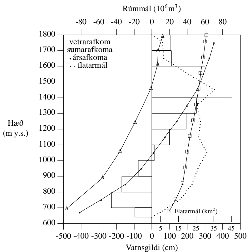
Mynd V-2. Línurit yfir afkomu Þjórsárjökuls í Hofsjökli 1992-1993.
