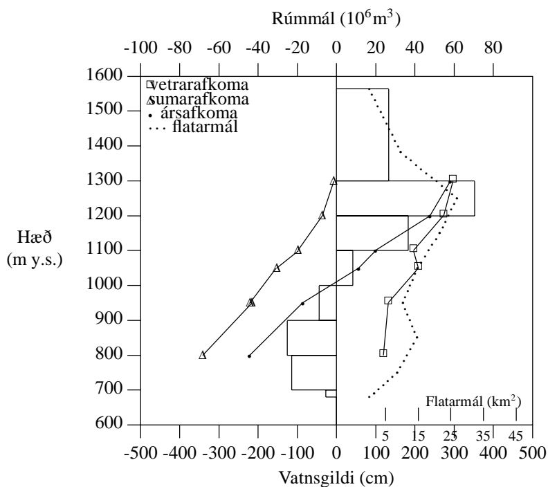
Mynd V-16. Línurit yfir afkomu Eyjabakkajökuls í Vatnajökli 1992-1993.
