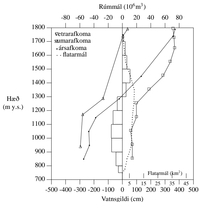
Mynd V-6. Línurit yfir afkomu Blágnjúpukuls í Hofsjökli 1993-1994.
