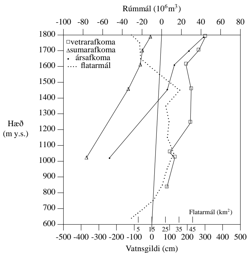
Mynd V-11. Línurit yfir afkomu Þjórsárjökuls í Hofsjökli 1995-1996.
