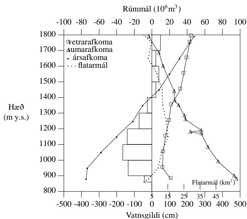
Mynd V-13. Línurit yfir afkomu Sátujökuls í Hofsjökli 1996-1997.
