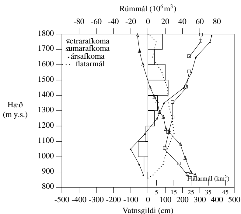
Mynd V-1. Línurit yfir afkomu Sátujökuls í Hofsjökli 1992-1993.
