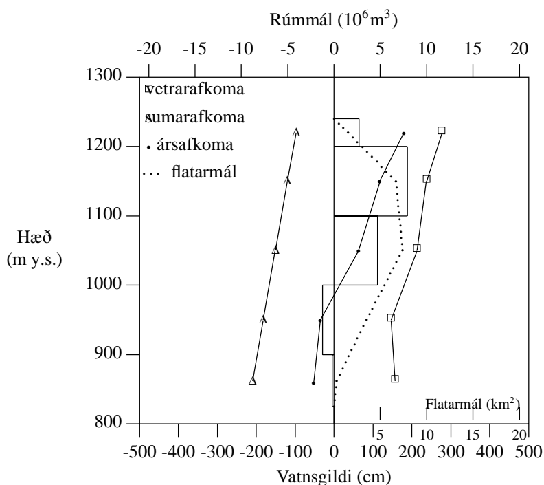
Mynd V-19. Línurit yfir afkomu Þrándarjökuls 1992-1993.
