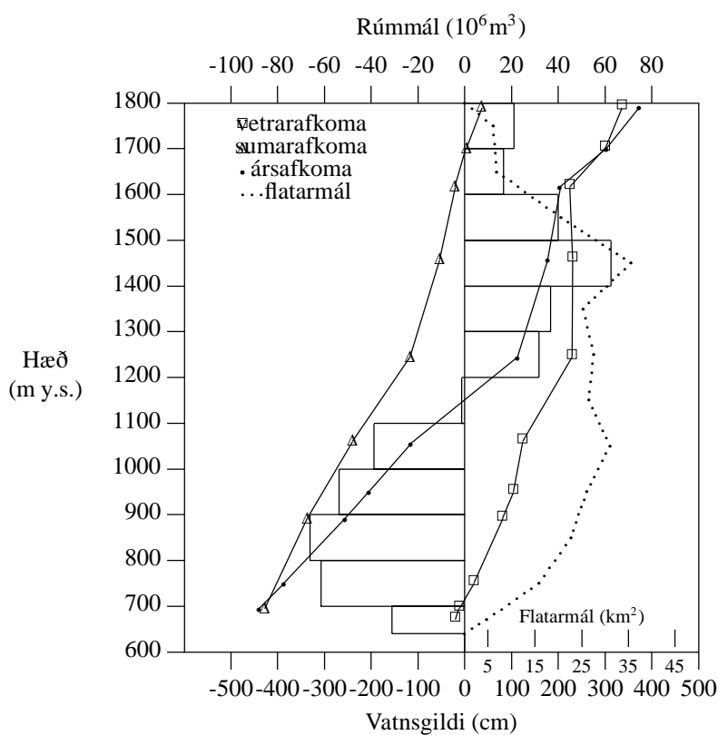
Mynd V-5. Línurit yfir afkomu Þjórsárjökuls í Hofsjökli 1993-1994.
