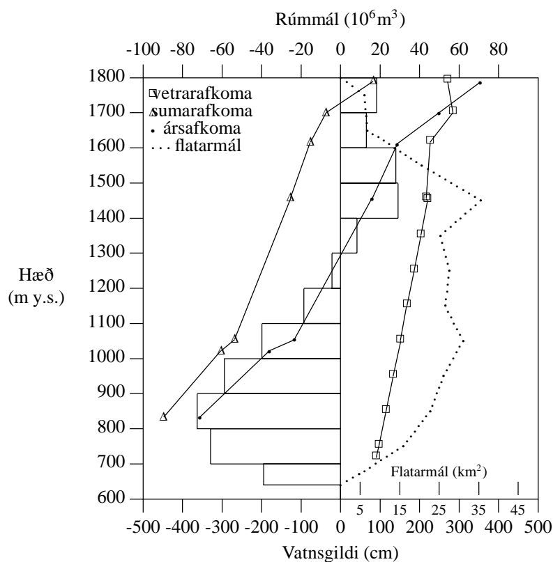
Mynd V-8. Línurit yfir afkomu Þjórsárjökuls í Hofsjökli 1994-1995.
