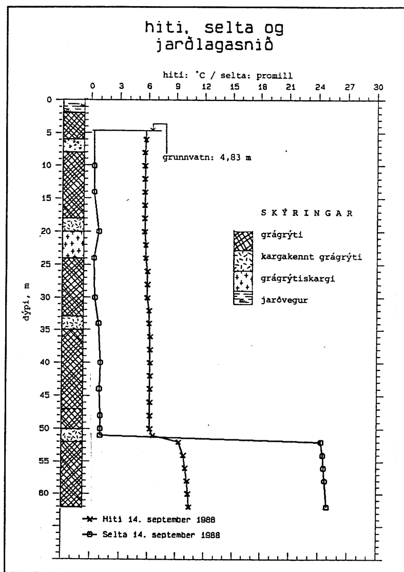
Mynd 2. Dæmigerð jarðlagaskipan á Romshvalanesi
