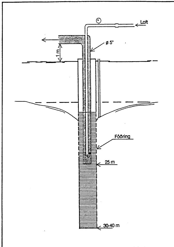
Mynd 4. Loftdæling
