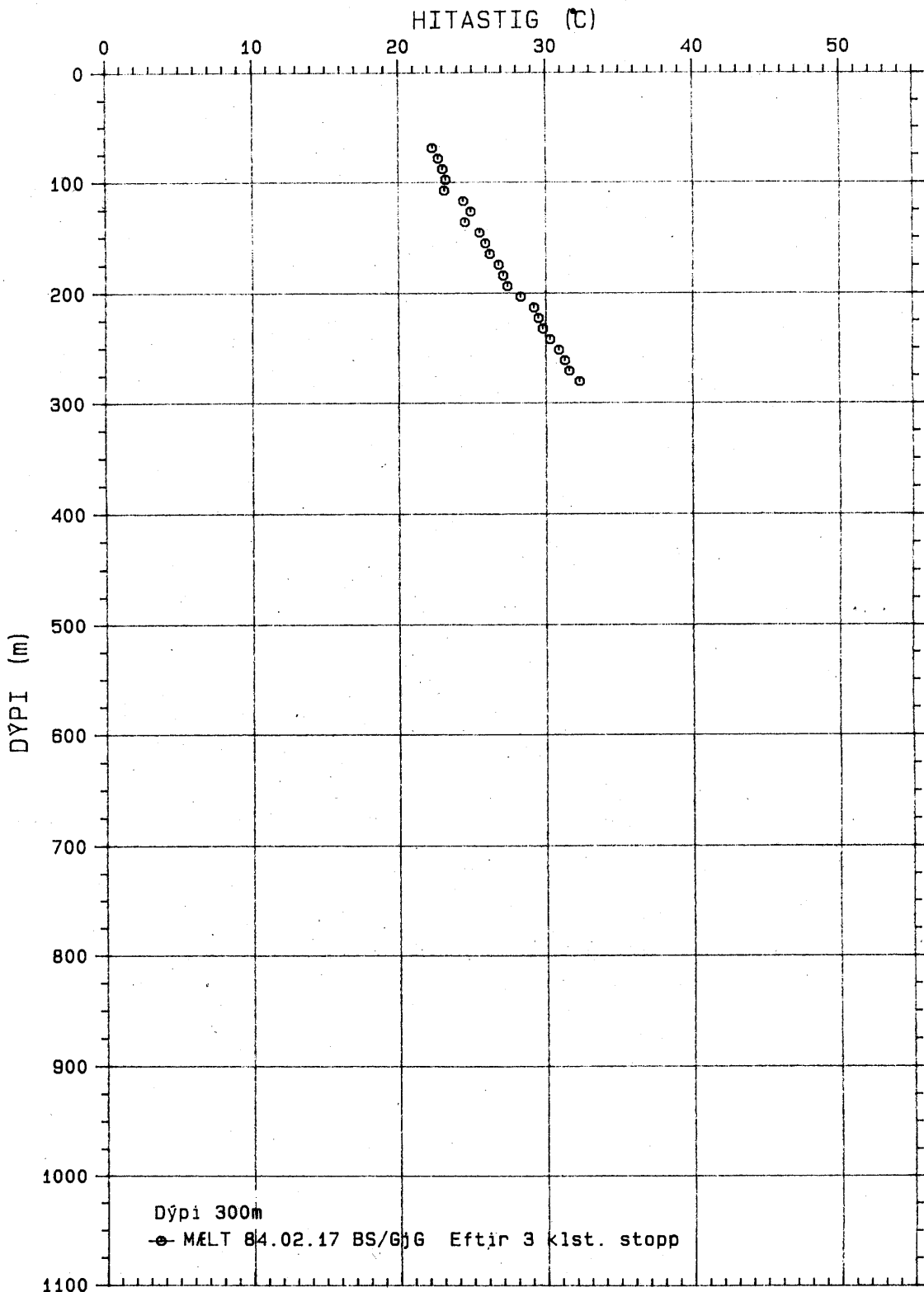
Mynd 8 Hitamæling 84.02.17
