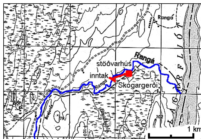
Mynd 15: Mögulegt fyrirkomulag virkjunar í Rangá
