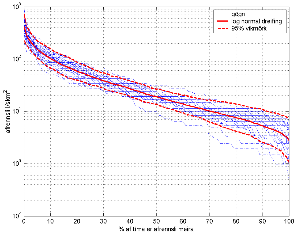
Mynd 14: Langæislína Miðhúsaár, vhm 47. Afrennsli skv. mælingum 1949 – 1989
