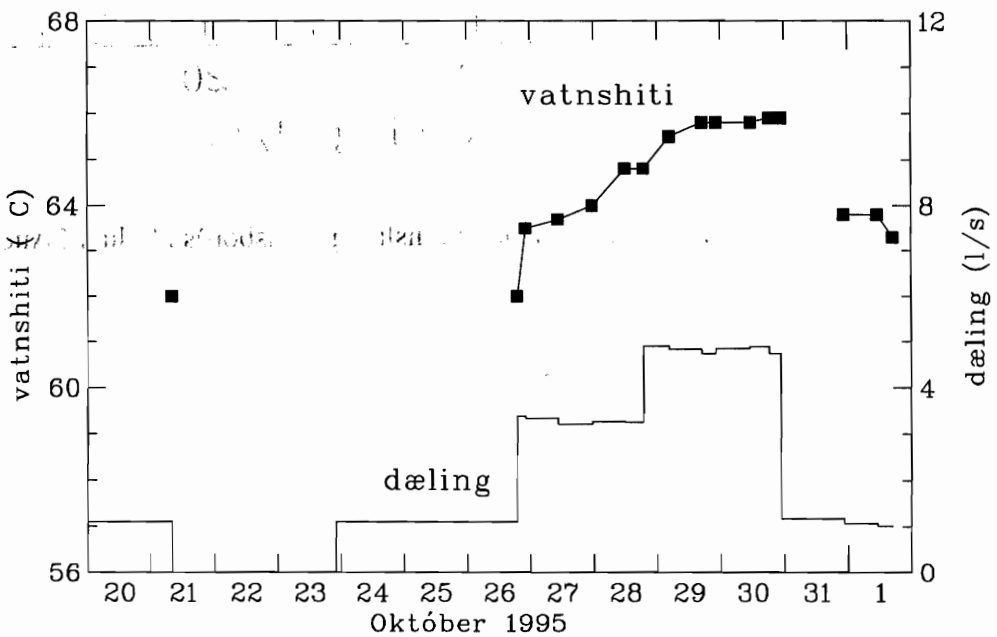
Mynd 2. Vatnshiti og vinnsla í prófun holu 4 í Auðsholti.
