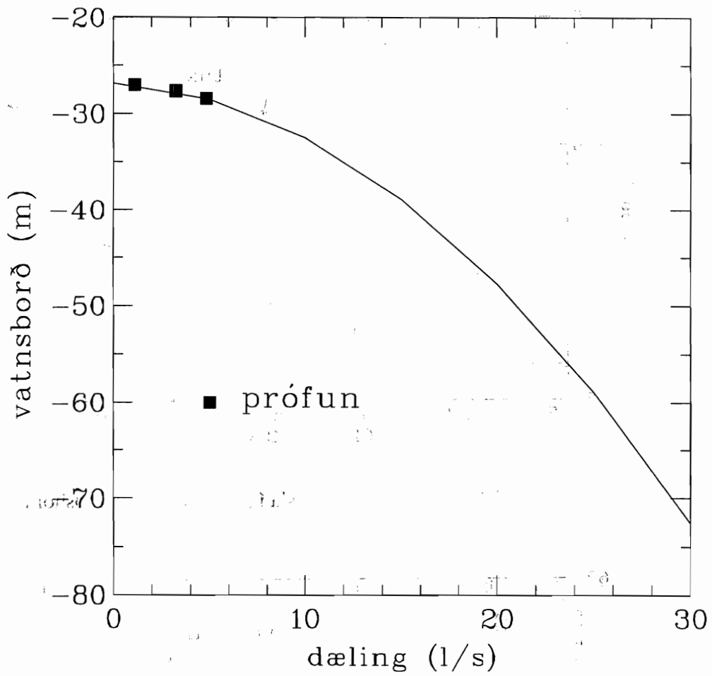
Mynd 3. Áætlað samband vinnslu og vatnsborðs í holu 4 í Auðsholti.
