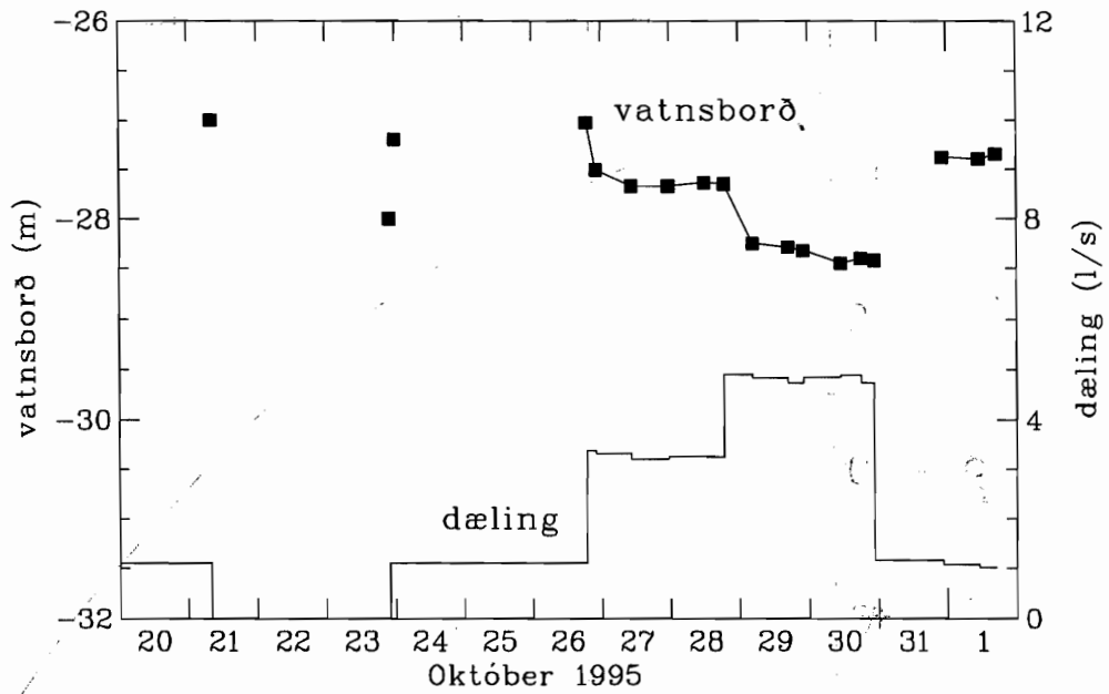
Mynd 1. Vatnsborð og vinnsla í prófun holu 4 í Auðsholti.
